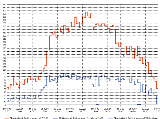
Příklad profilu zatížení za 24 hodin
